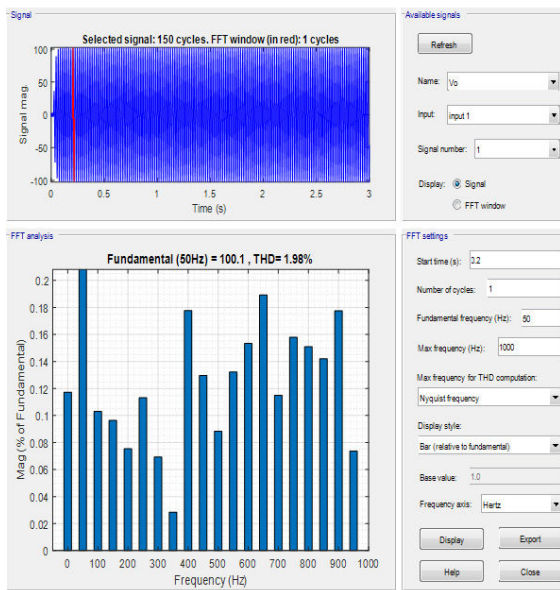
Fig.9. THD values.
